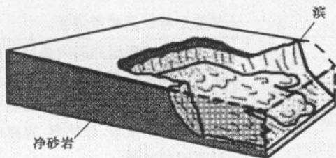
(g) 流动(Flow)
