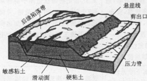
(e) 滑动(Slide)
