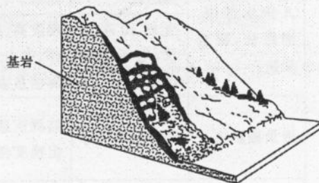
(d) 滑动(Slide)
