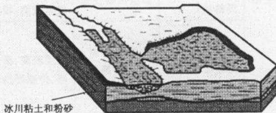
(h) 流动(Flow)
